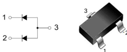
SOT - 23
