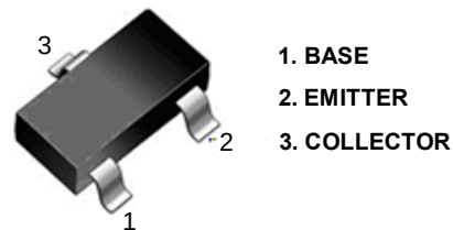
SOT - 23
